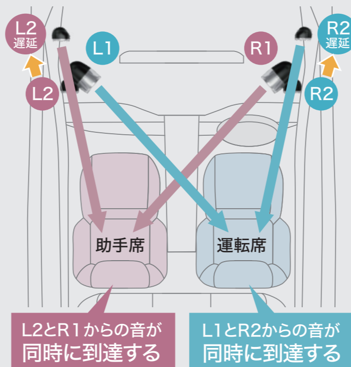
左右席同時定位原理図
