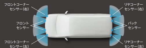
センサーイメージ図
