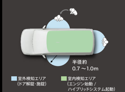
スマートエントリーシステム検知エリア
