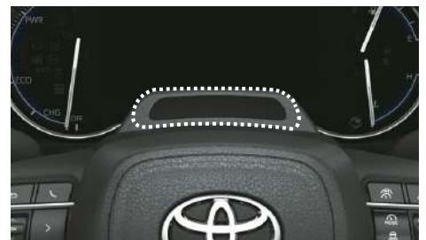
ドライバーモニターカメラ ■ドライバーモニターカメラで運転者の顔の位置・向きや眼の開閉状態を検知。運転者が周囲の状況を確認し運転操作できる状態であるかシステムが判断し、プザーとディスプレイ表示で注意喚起を行います。*3
