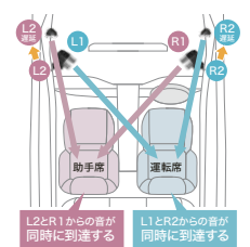
左右席同時定位原理図
