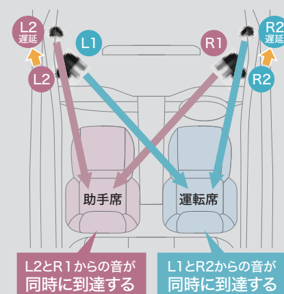
左右席同時定位原理図
