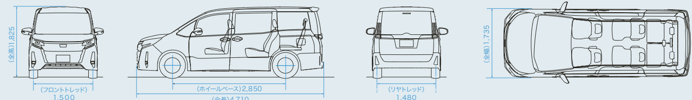
寸法図:トヨタ ノア Si(7人乗り・2WD) 単位:mm
