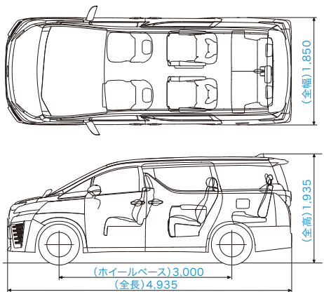
■寸法図(単位:mm) ZG(7人乗り・2WD)
