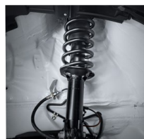
マクファーソンストラット式 フロントコイルサスペンション
